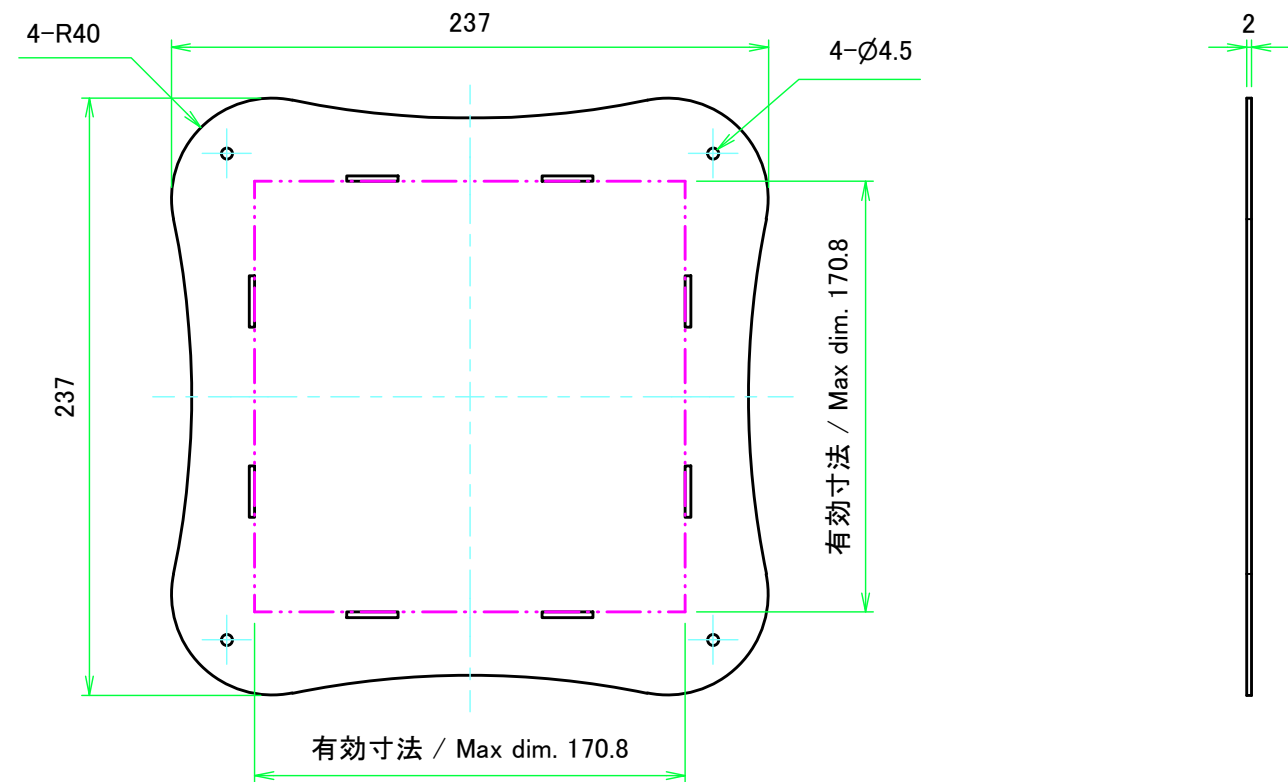
上カバー表面 / Top cover Frontside
