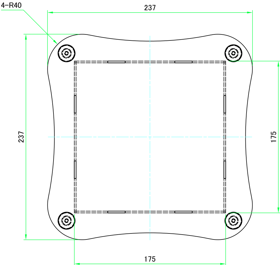
上カバー / Top cover
