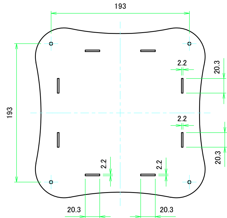
上カバー裏面 / Top cover Backside
