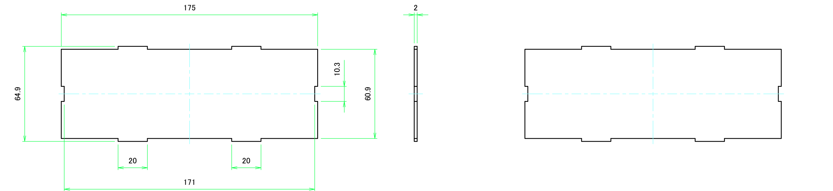
Wパネル1表面 / W Panel 1 Frontside
