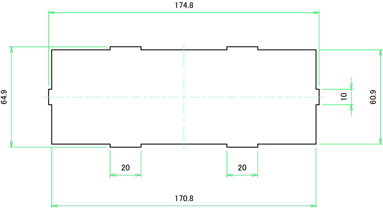
Dパネル1表面 / D Panel 1 Frontside
